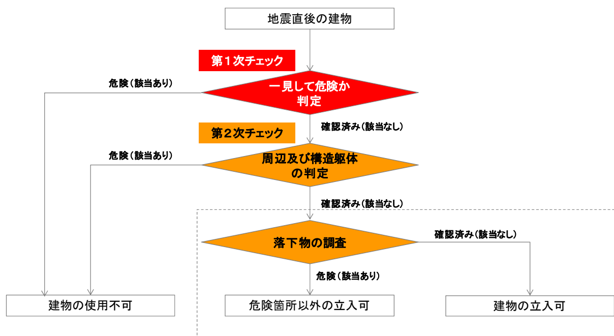
図表 鉄骨造の建物の安全確認の流れ
