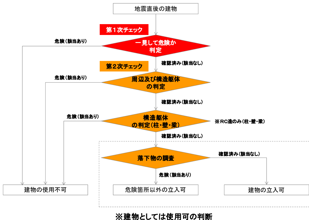
図表 鉄筋コンクリート造の建物の安全確認の流れ
