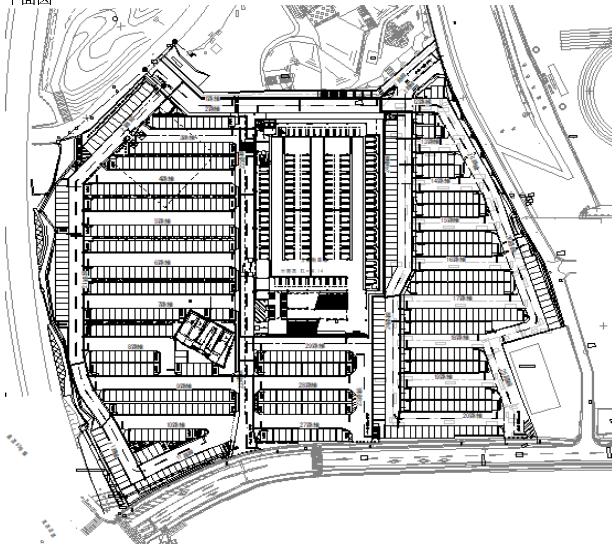
コザ運動公園立体駐車場 平面図
