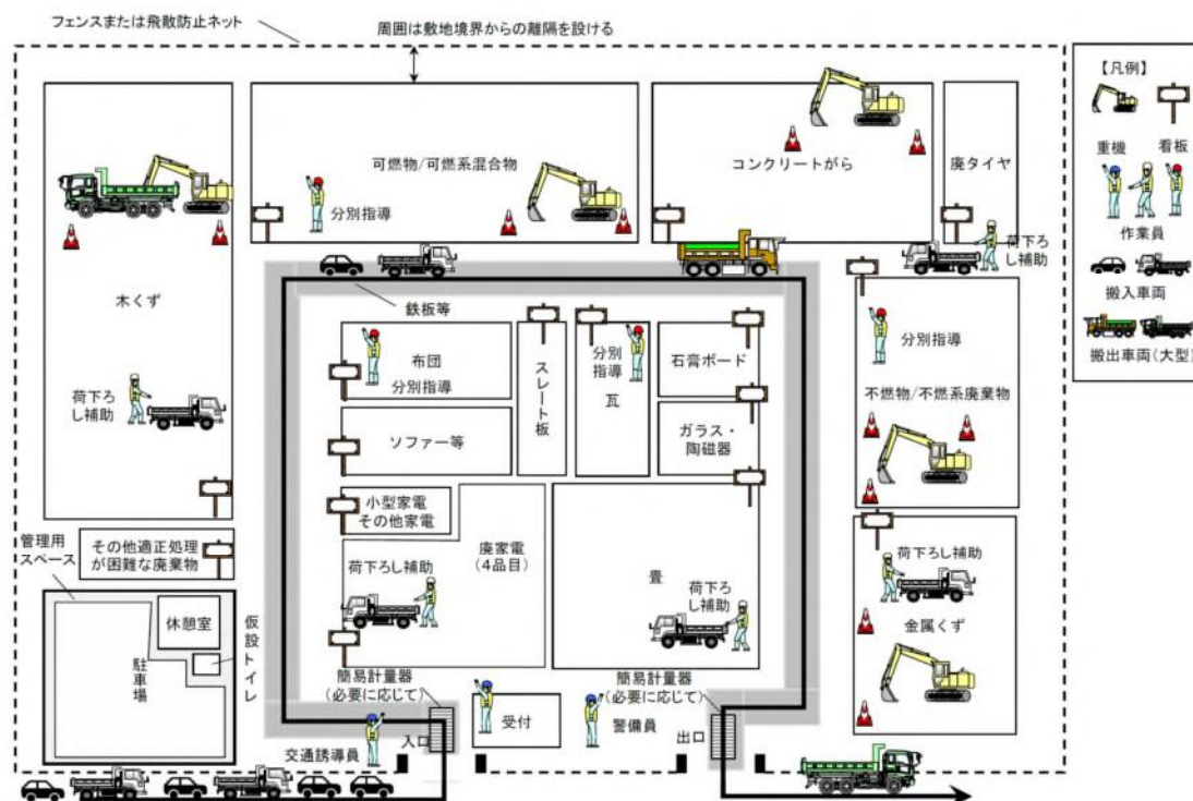
図2-6-5 一次仮置場の配置計画（例）
