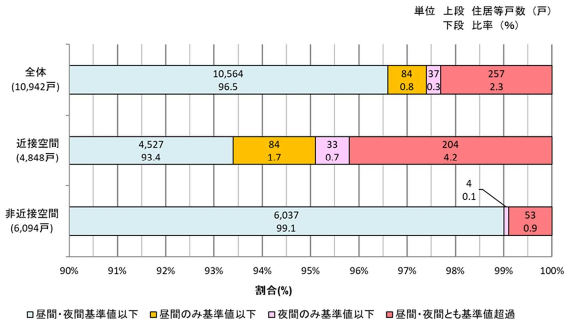
図.4 全体および近接空間・非近接空間における環境基準の達成状況
